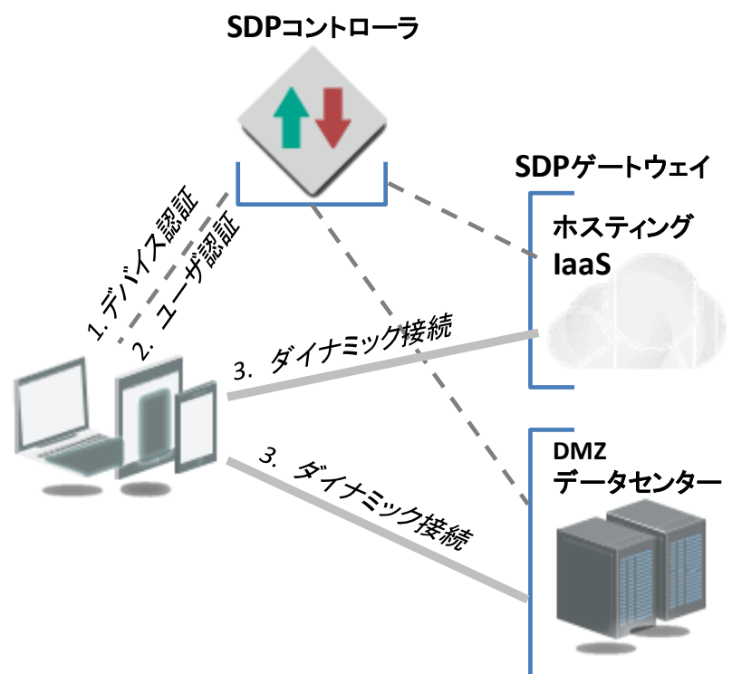
SDP通信ダイアグラム
